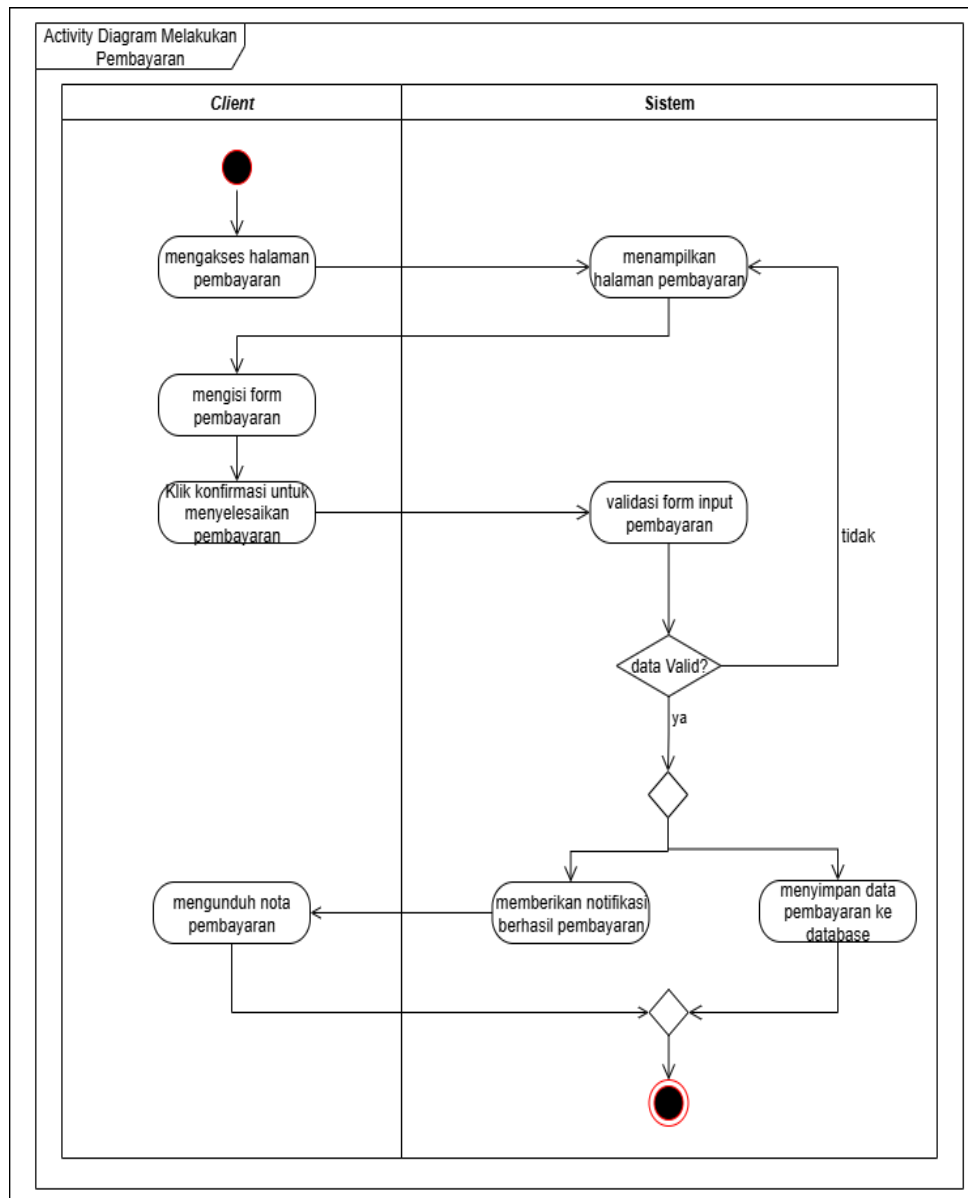
Gambar III.7 Activity Diagram Client Melakukan Pembayaran
