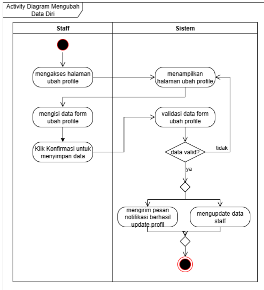
Gambar III.11 Activity Diagram Staff Mengubah Data Diri
