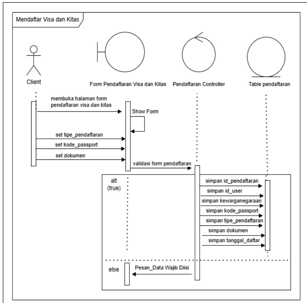
Gambar III.29 Sequence Diagram Client Melakukan Pendaftaran Visa
