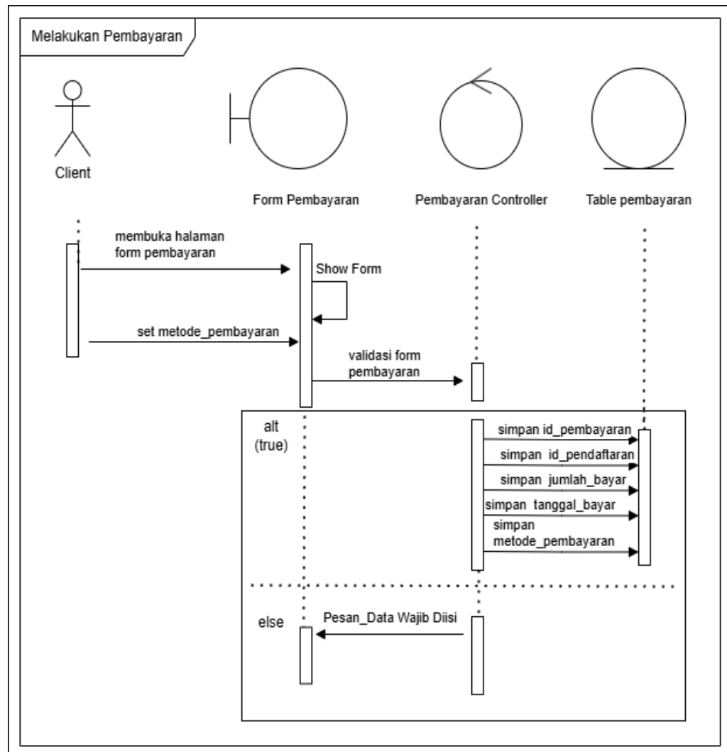
Gambar III.31 Sequence Diagram Client Melakukan Pembayaran
