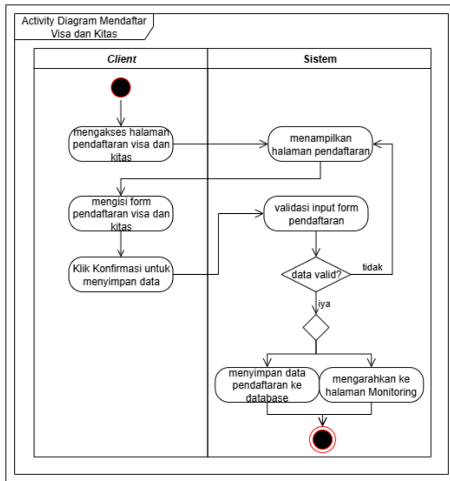
Gambar III.5 Activity Diagram Client Mendaftar Visa dan KITAS
