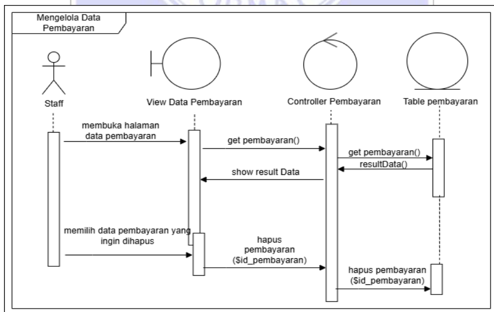
Gambar III.38 Sequence Diagram Staff Mengelola Data Pembayaran
