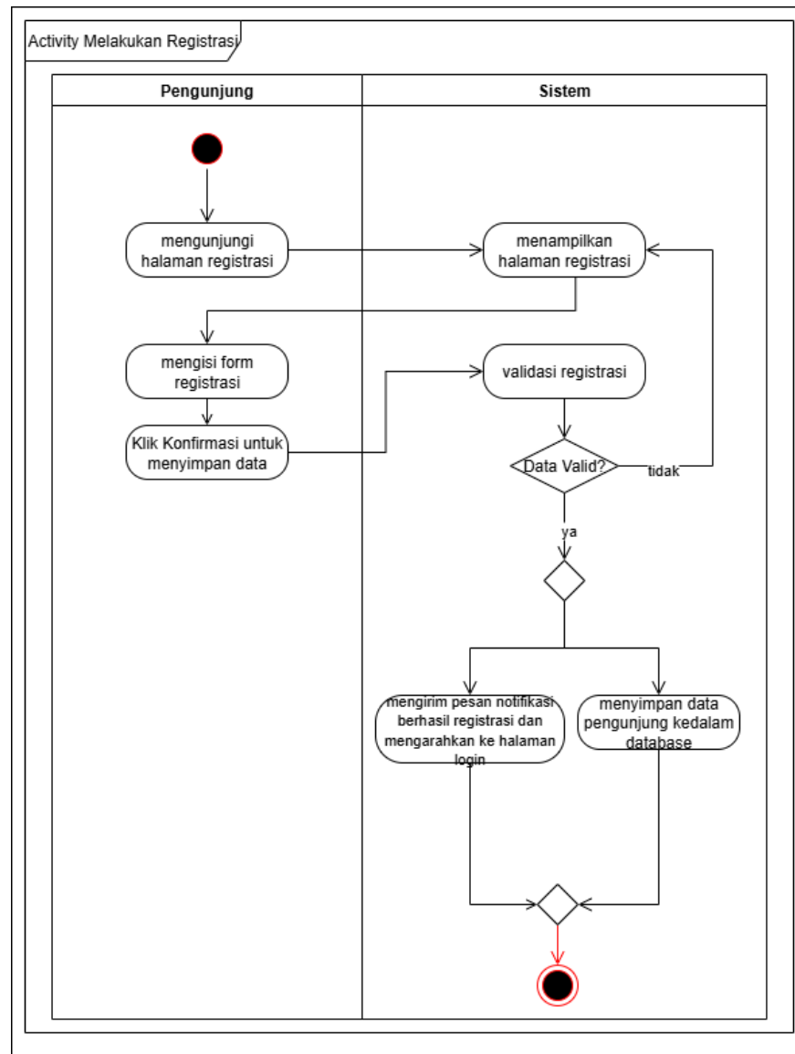
Gambar III.2 Activity Diagram Pengunjung Melakukan Registrasi
